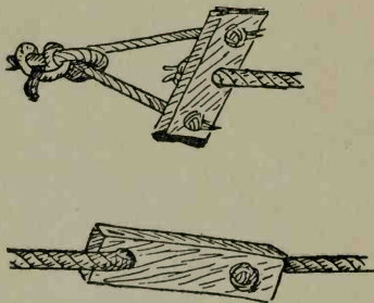
FIG. 145.—Swivels.
